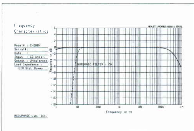
周波数特性
